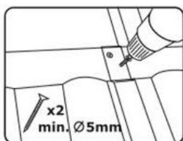
UKOTVIT DO LATĚ
